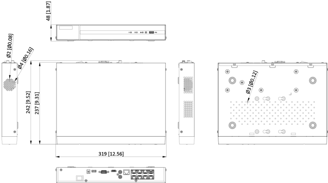
scale/1:1;Unit/mm
